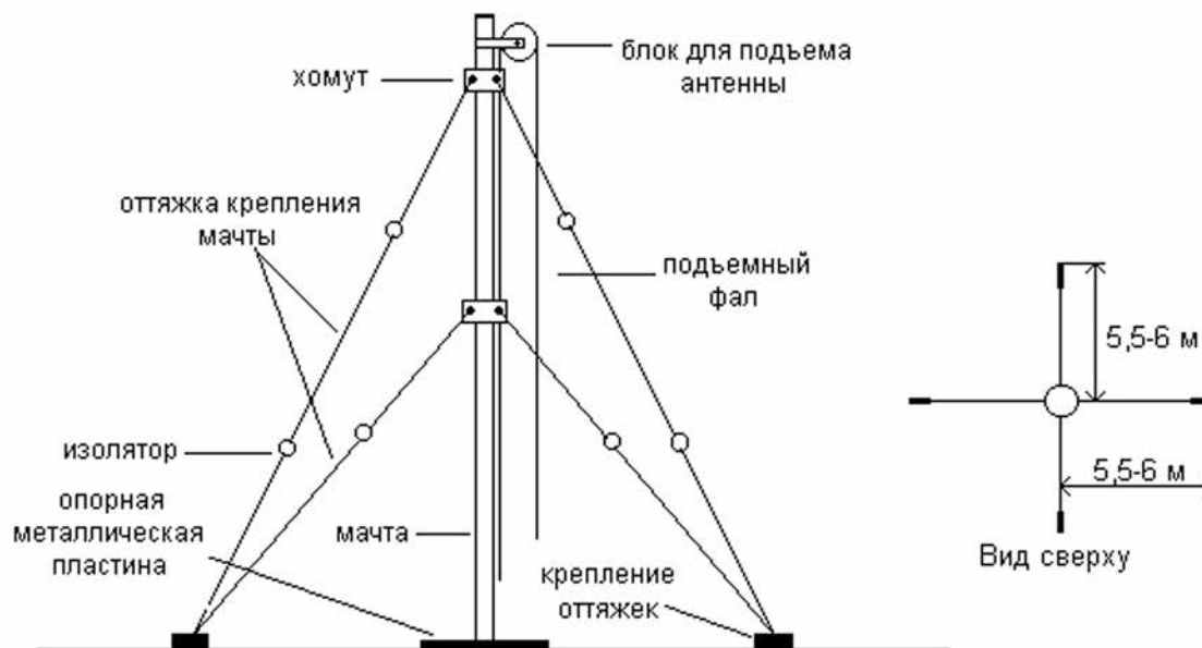
Рис. 2.11. Антенная мачта в развернутом виде
