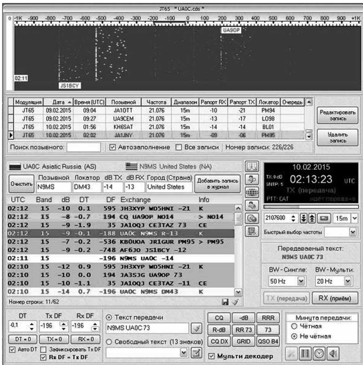
Рис. 9.5. Рабочее окно программы «KROT» для режима JT65A
