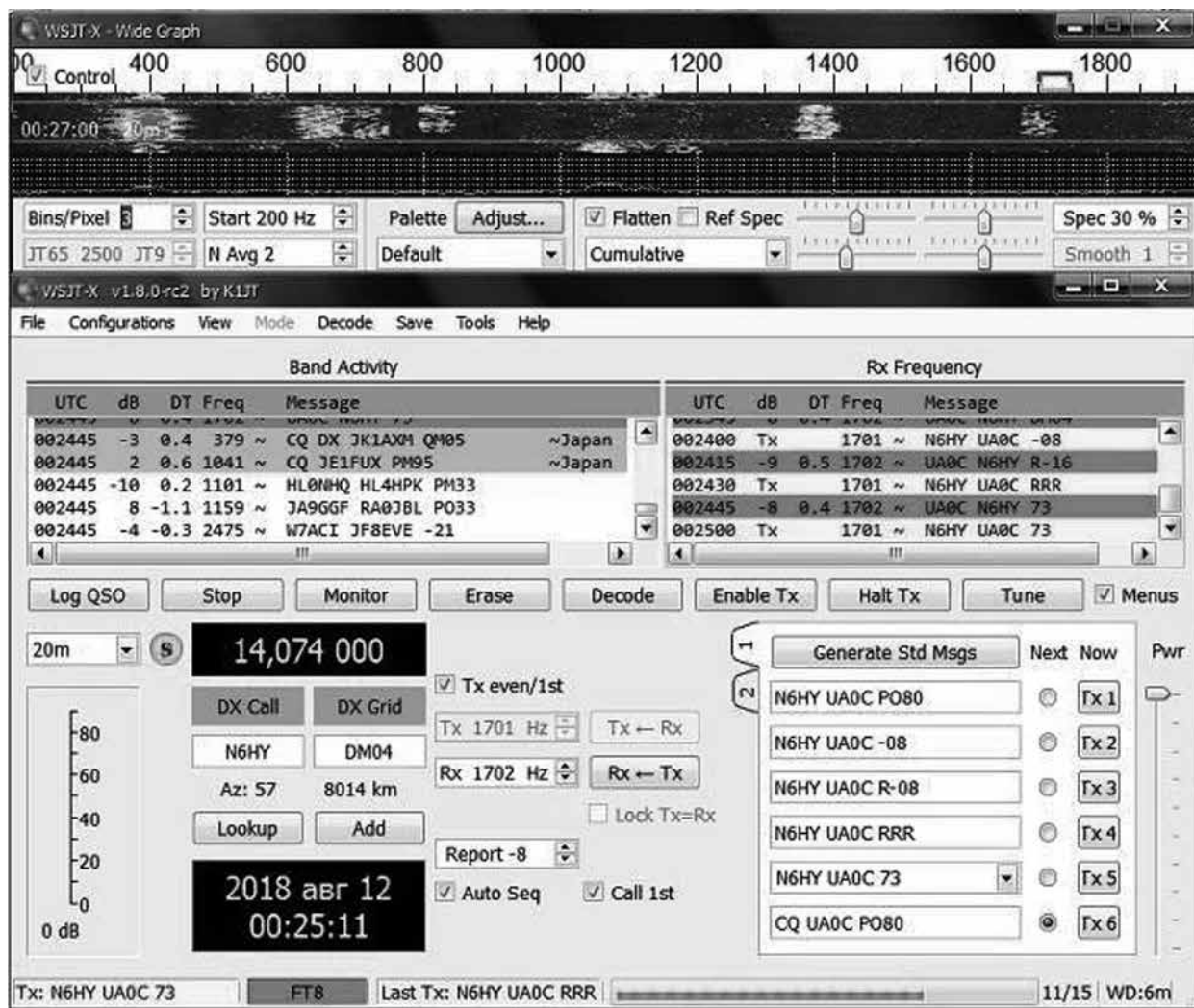
Рис. 9.7. Рабочие окна программы WSJT-X для режима FT8
