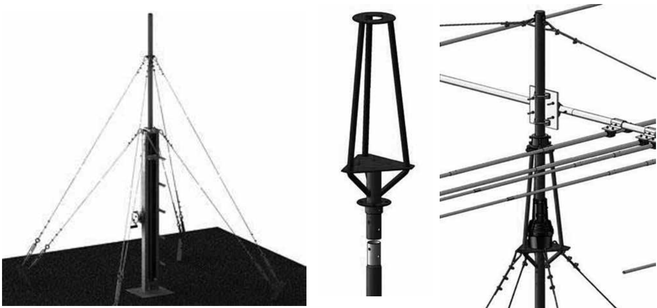
Рис. 2.12. Трубчатая мачта со станком-подъемником СТ-S1Т
