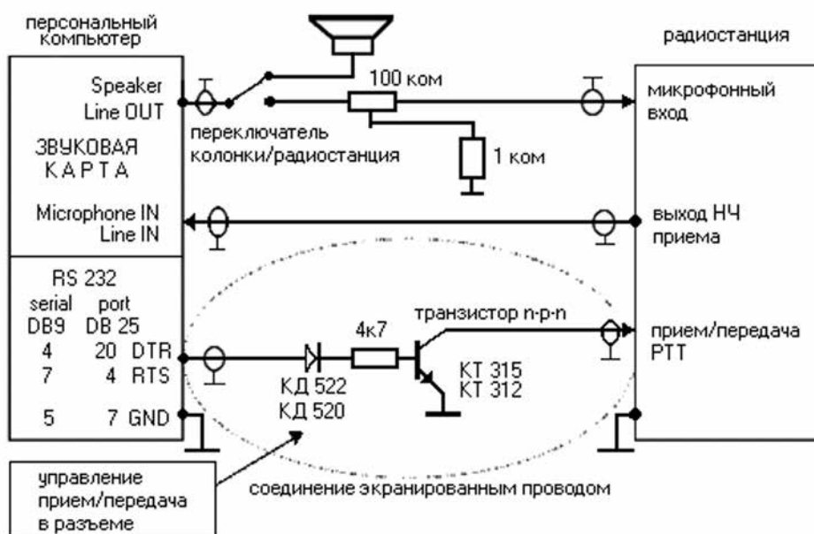
Рис. 9.1. Подключение «компьютер-трансивер»
