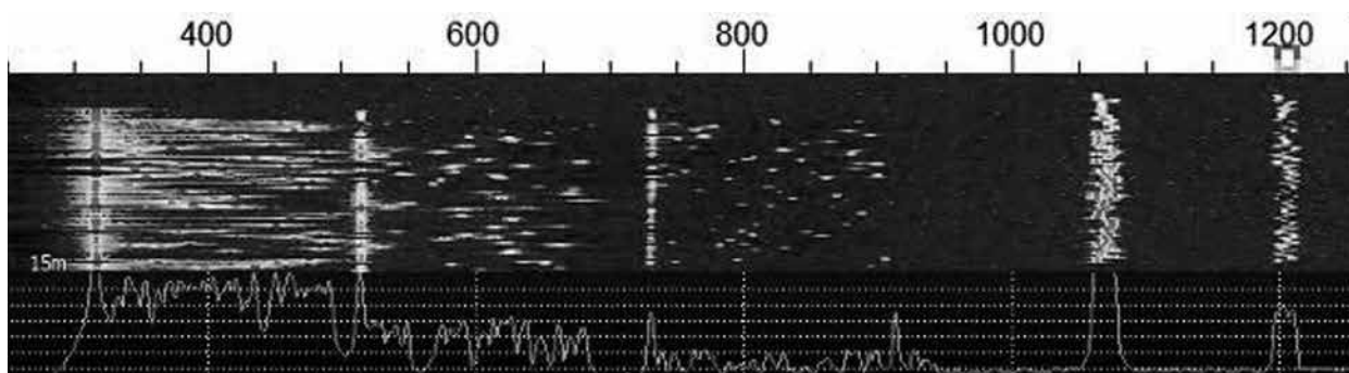
Рис. 9.6. Вид сигналов JT65A (три слева) и JT9 (два справа), принятых с использованием программы WSJT-X
