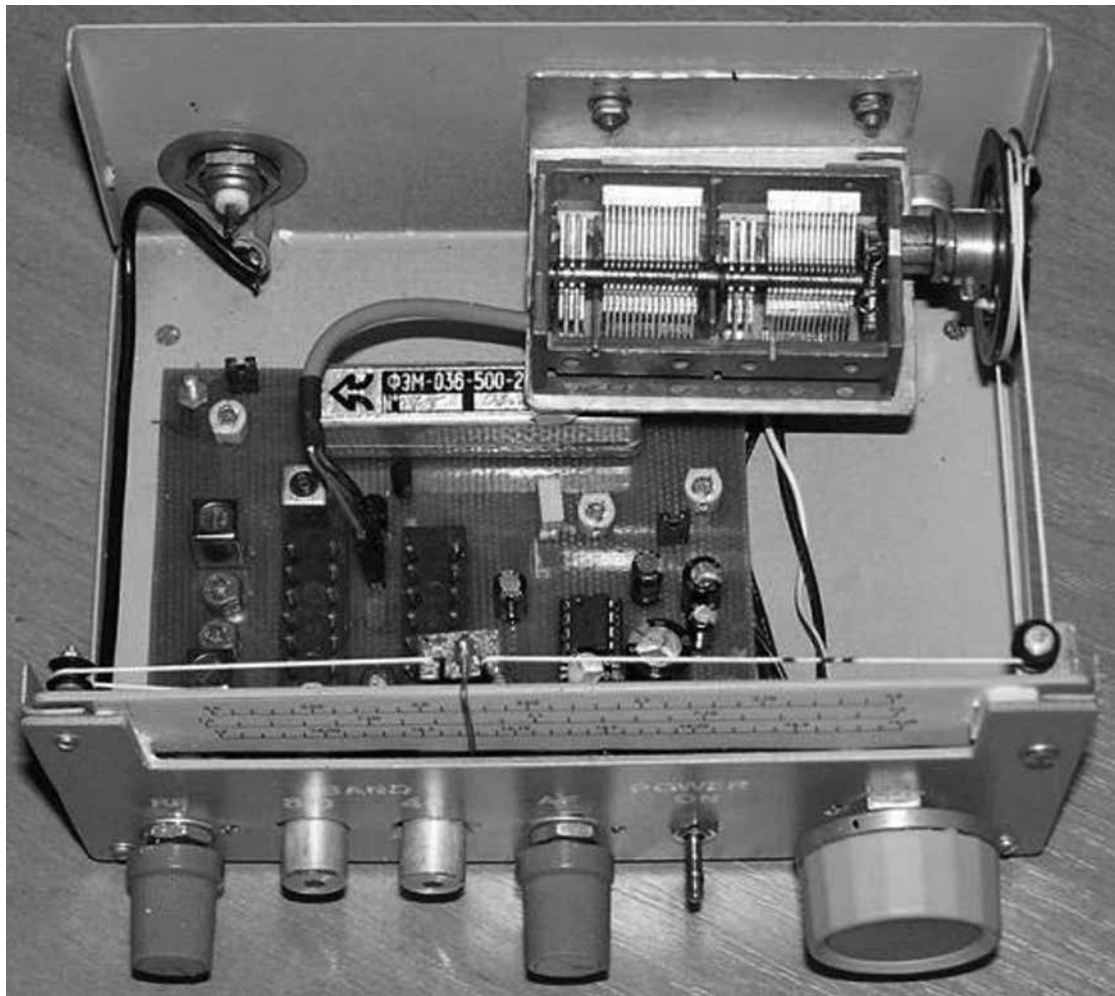
Рис. 2.9. Трехдиапазонный приёмник радиолюбителя-наблюдателя на диапазоны 20, 40 и 80 м.
