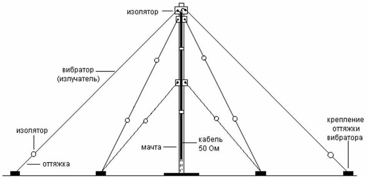
Рис. 2.14. Антенна «Inverted V»
