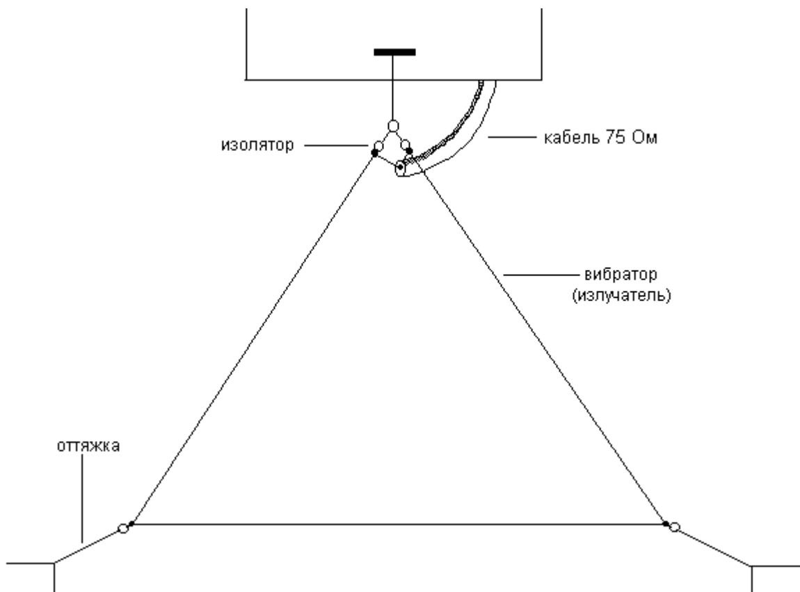
Рис. 2.15. Антенна «треугольник»
