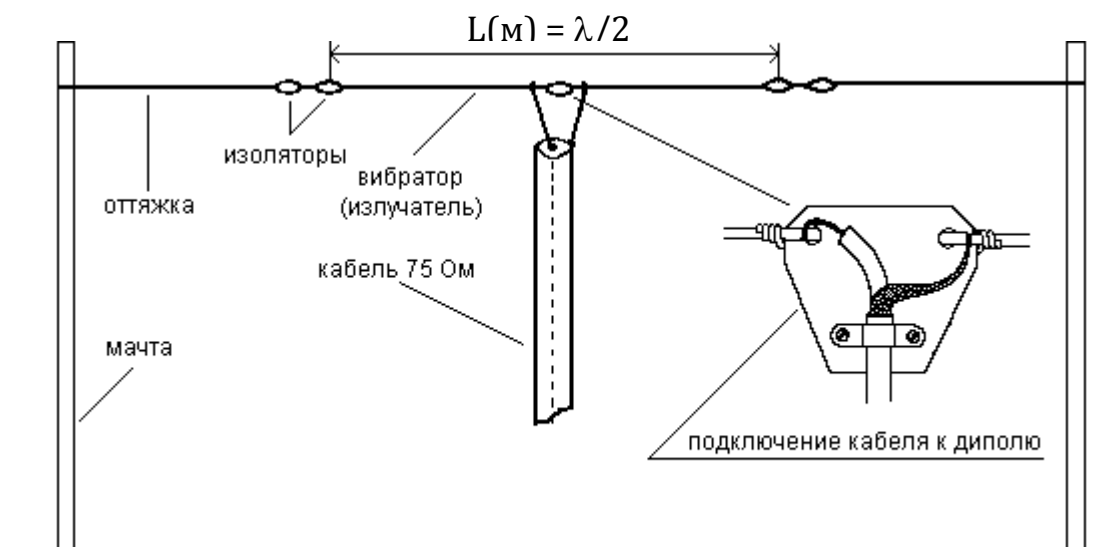
Рис. 2.13. Антенна «диполь»
