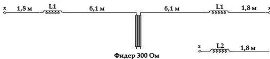
Рис. 2.17. Антенна «укороченный диполь»
