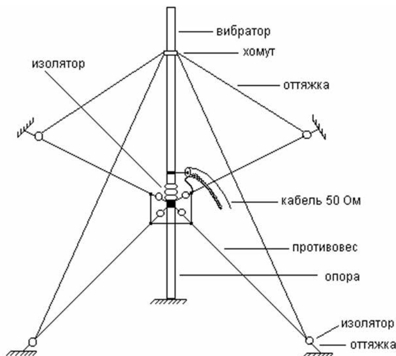
Рис. 2.16. Антенна «граунд-плэйн»
