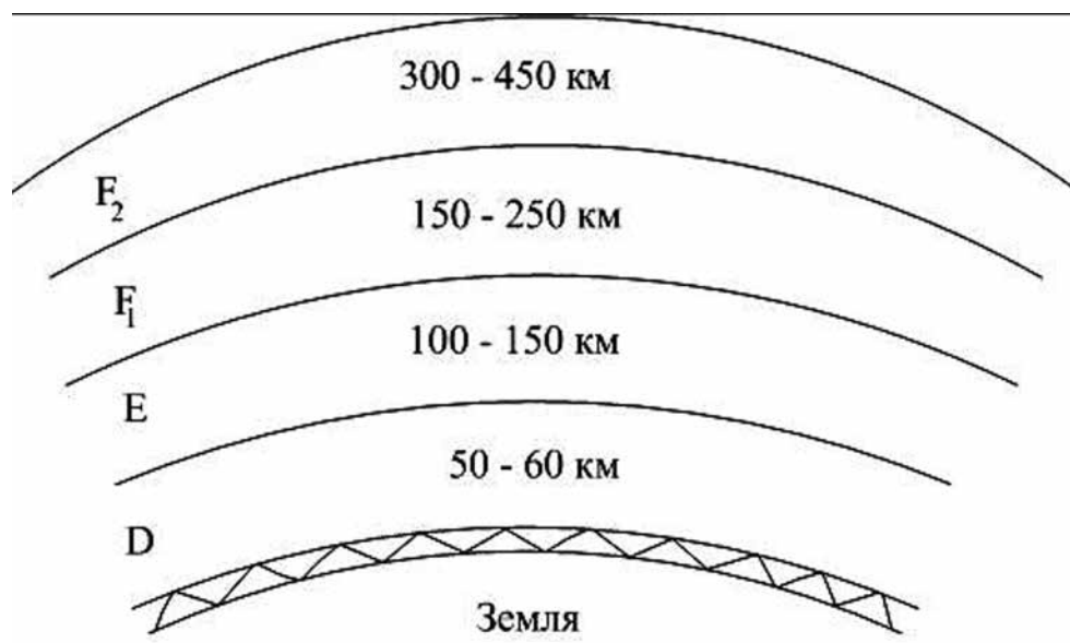
Рис. 2.2. Ионосферные слои
