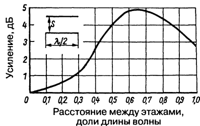
Рис. 13.5. Зависимость максимального усиления двух синфазных вибраторов, расположенных один над другим, от межэтажного промежутка S (по ARRL-Antennen Book)
