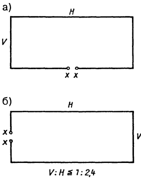
Рис. 15.5. Волновой прямоугольник: а – горизонтально поляризованный; б – вертикально поляризованный
