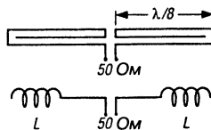
Рис. 10.28. Принцип действия двухдиапазонной антенны Mop-Gain в 80-метровом диапазоне
