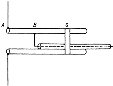
Рис. 7.22. Шлейф Пози
