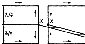
Рис. 13.14. Синфазная горизонтальная антенна с центральным питанием
