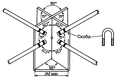
Рис. 18.50. Крепление кронштейнов
