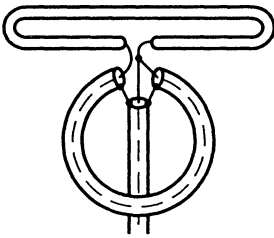
Рис. 7.13. Реализация полуволновой петли
