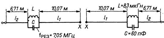
Рис. 10.22. Антенна W3DZZ
