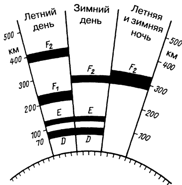
Рис. 2.2. Слои ионосферы
