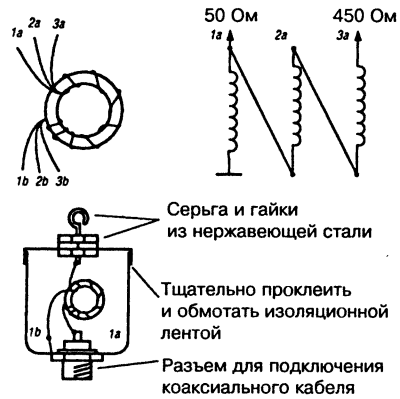
Рис. 6.28. Устройство и схема широкополосного трансформатора
