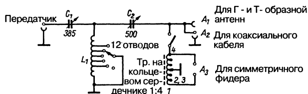
Рис. 8.16. Т-образный СЛП
