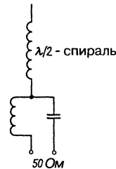
Рис. 19.85. Принципиальная схема согласования КВ спиральной антенны
