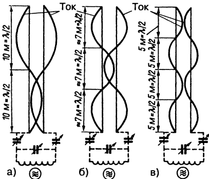
Рис. 18.1. Двухпроводная линия длиной 20 м: а – при возбуждении двумя половолнами ( \lambda \approx 20 м); б – тремя половолнами ( \lambda \approx 15 м); в – четырьмя половолнами ( \lambda \approx 10 м)
