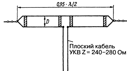
Рис. 10.4. Петлевой вибратор в качестве КВ антенны
