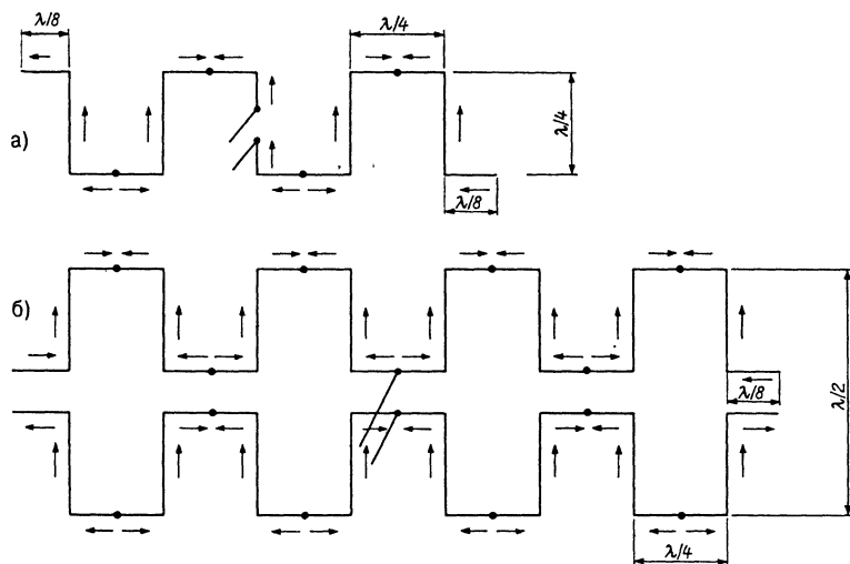
Рис. 13.22. Антенны Брюса: а – простая, б – двойная
