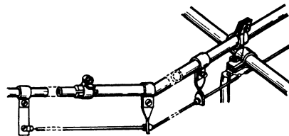
Рис. 15.22. Конструкция гамма-согласователя
