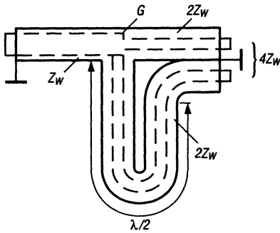
Рис. 7.12. Принцип действия полуволнового шлейфа
