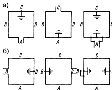
Рис. 15.3. Поляризация и возможности заземления квадратной рамки:
